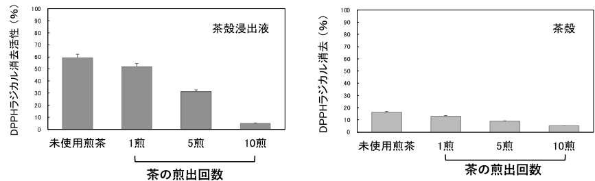
(図) 乳酸発酵1週間後の茶殻浸出液と茶殻の抗酸化活性 (平均値±標準誤差, n=3)
